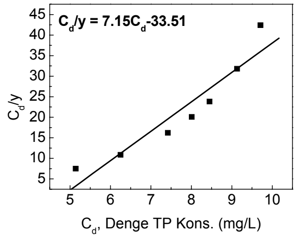
Şekil 7. Cüruf için 4 °C'de Langmuir izotermini
