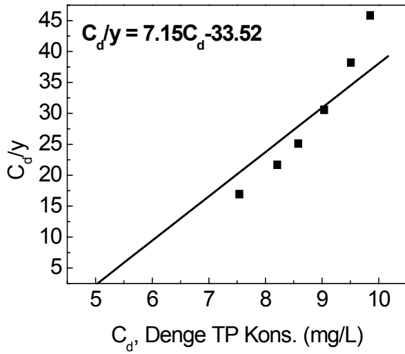
Şekil 9. Çakıl için 4 °C'de Langmuir izotermi
