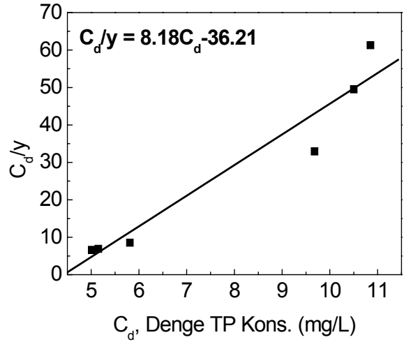
Şekil 6. Cüruf için 21 °C'de Langmuir izotermini
