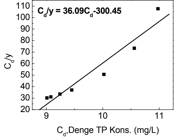
Şekil 5. Perlit için 4 °C 'deLangmuir izotermini
