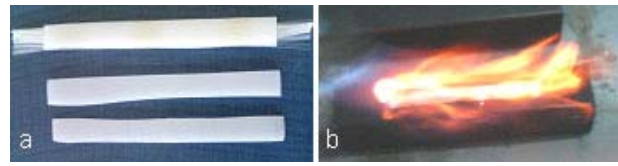
Şekil 3. Polietilen lifli, liffsiz numuneler(a) ve direkt alev uygulaması (b)
