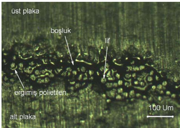
Şekil 12. Aşama III 'de endirekt ısıtılmış yoğun lifli numunedeki içyapı
