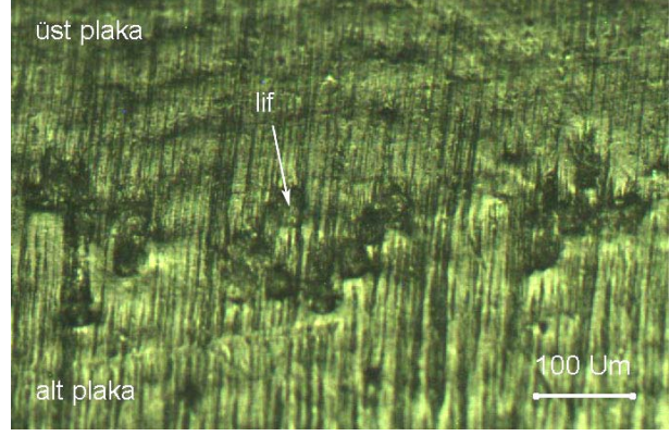
Şekil 13. Aşama III 'de endirekt ısıtılmış azaltılmış lifli numunedeki içyapı
