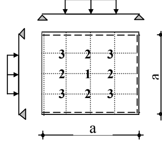
Şekil 5. Orta alanda q düzgün yayılı yük taşıyan 4 kenarı basit mesnetli plak
