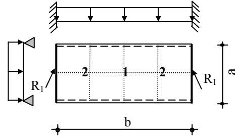
Şekil 7. İki karşılıklı kenarından basit mesnetli, diğer kenarlarından ankastre plak b/a=2
