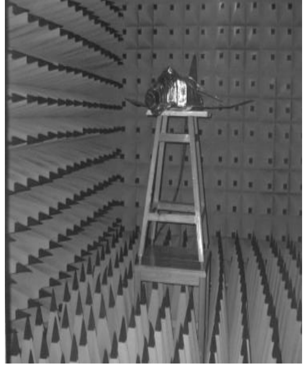
Şekil 9. Ölçekli model yansız ölçüm odasında
