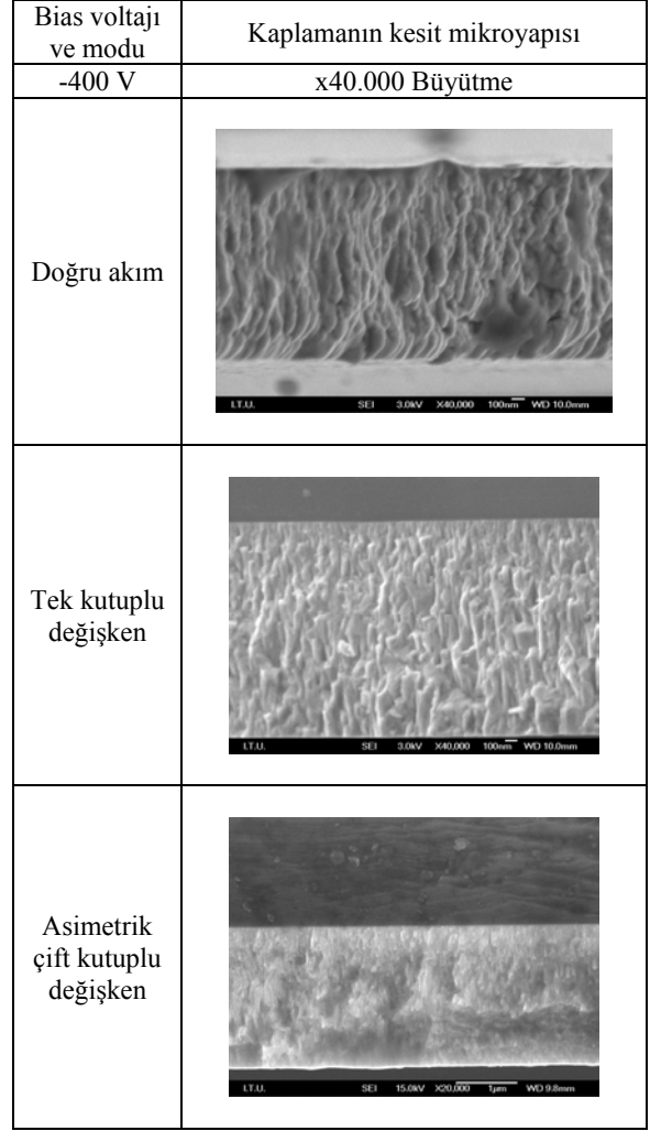
Şekil 7. -400 voltta değişik bias voltaj modlarında üretilen kaplamaların kesit mikroyapılarının kırık yüzey SEM fotoğrafları
