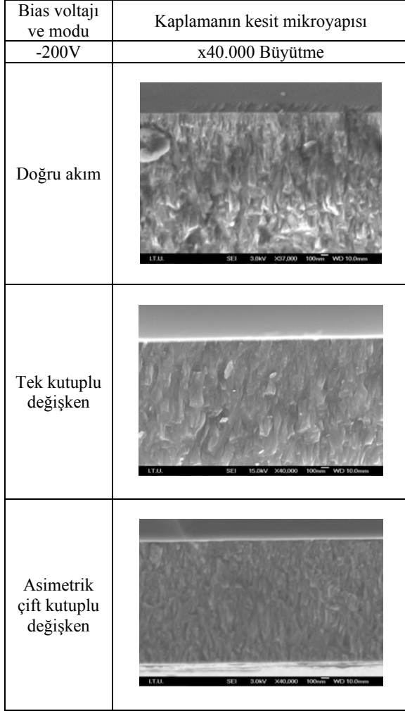
Şekil 6. -200 voltta değişik bias voltaj modlarında üretilen kaplamaların kesit mikroyapılarının kırık yüzey SEM fotoğrafları
