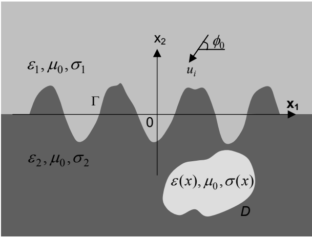
Şekil 1. Problemin geometrisi
