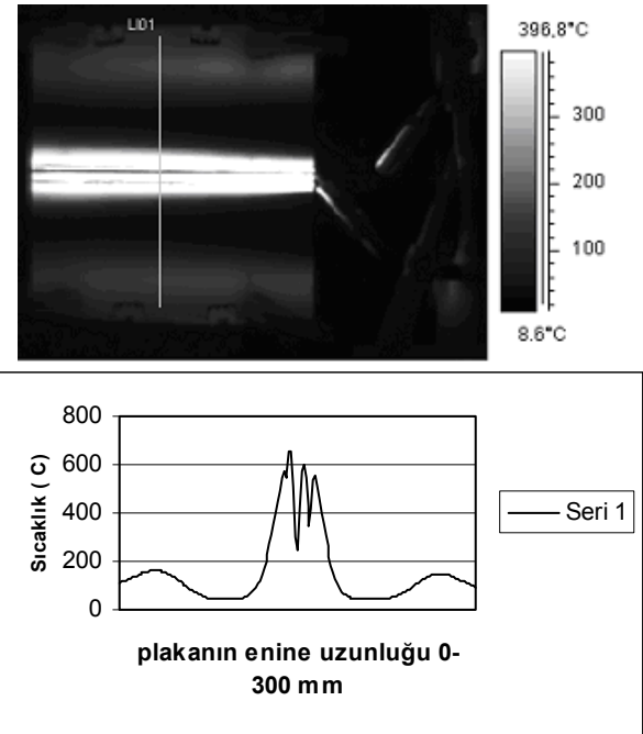
Şekil 9. Kaynak sonrası soğuma periyodunda LI01 kesiti boyunca sıcaklık dağılımı
