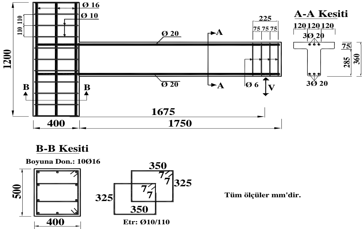
Şekil 1. Deney kirişlerinin donatı şeması
