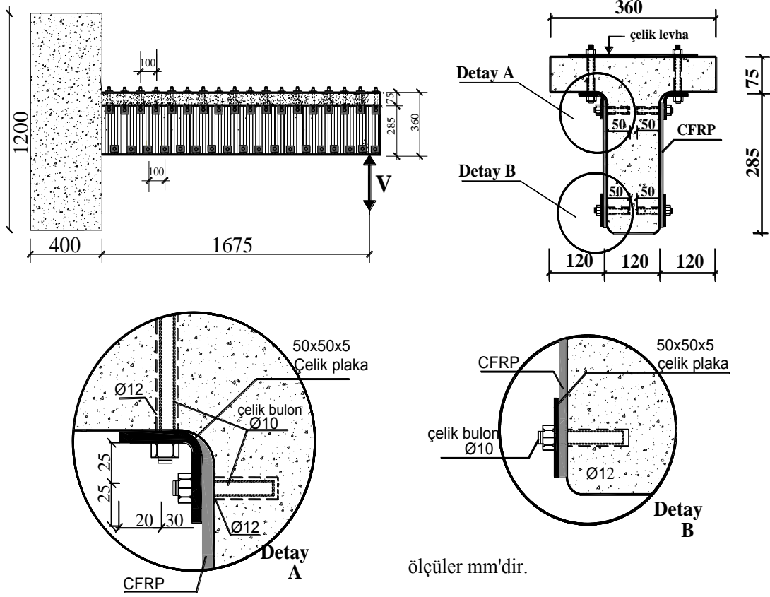
Şekil 2. Deneysel kirişlerinin CFRP düzenlemesi ve ankraj detayları
