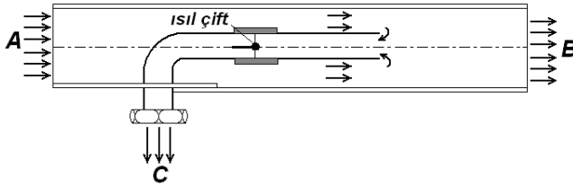
Şekil 5. Kuru ve yaş termometre sıcaklıklarını ölçmek için hazırlanan düzenele
