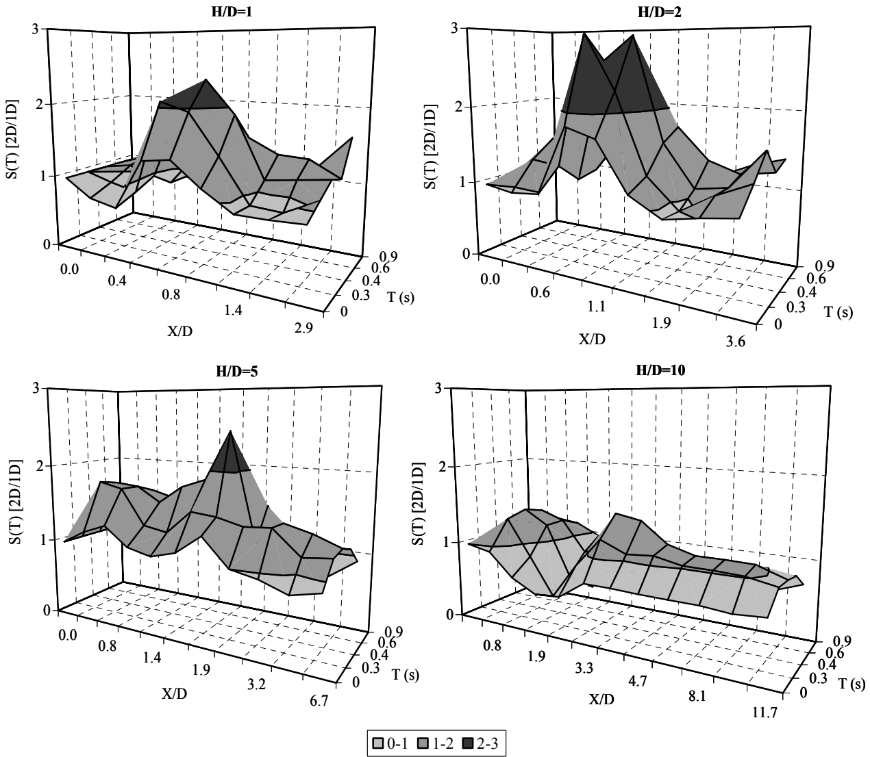
Şekil 8. Ova modellerinde 2D/1D şiddet faktörlerinin X/D ve periyota bağılı deęişimi
