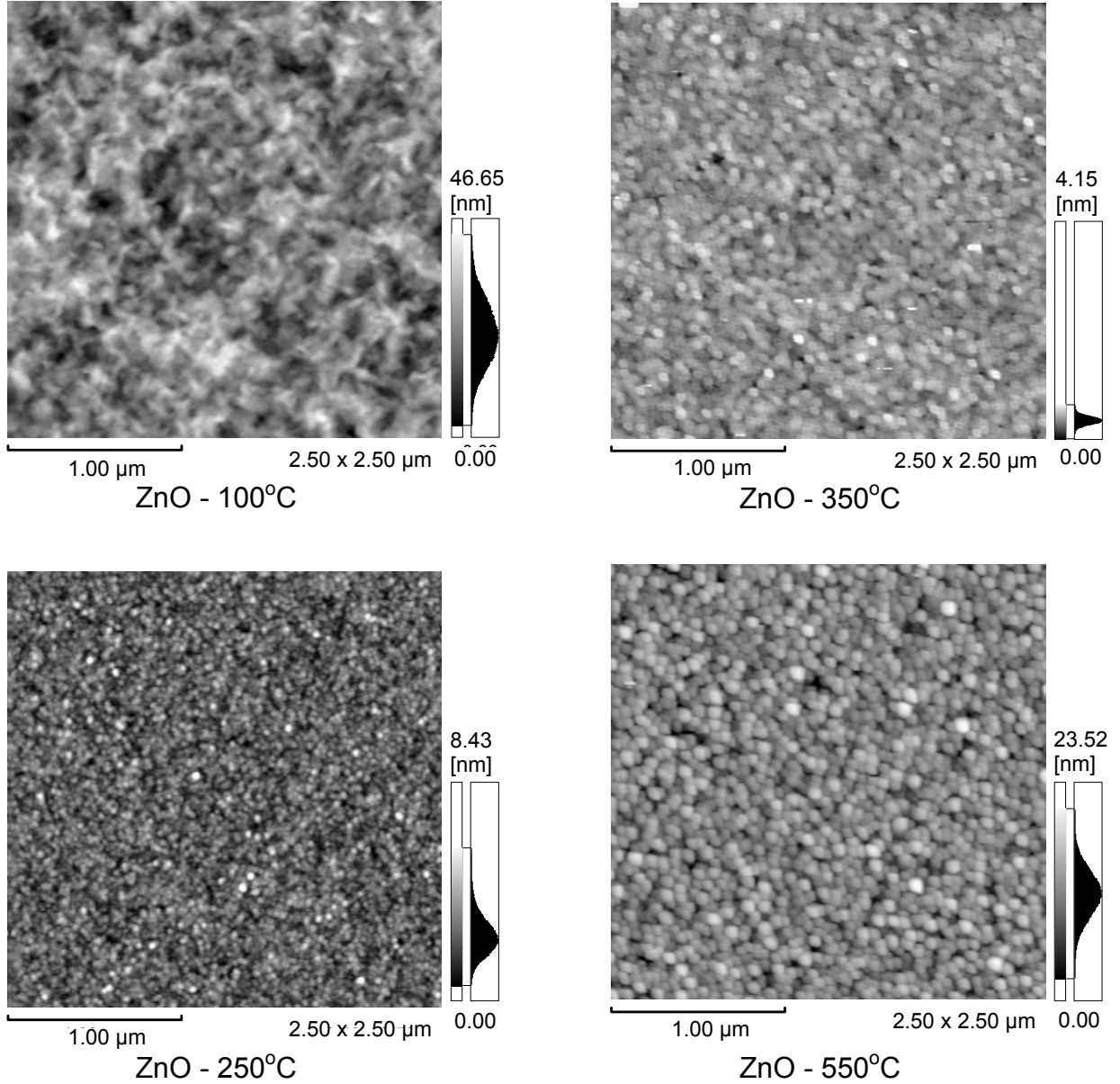
Şekil 4. Farklı sıcaklıklarda 1 saat ısıl işlem uygulanan ZnO filmlerinin AFM resimleri
