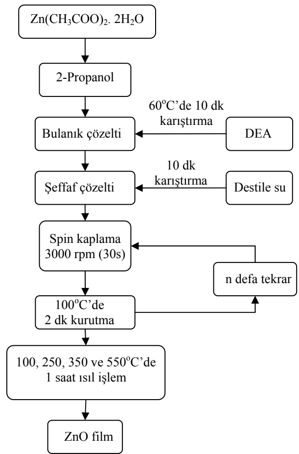
Şekil 1. ZnO ince filmlerin hazırlanma aşamaları
