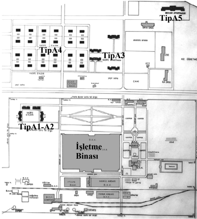
Şekil 2. Sümerbank Kayseri bez fabrikası ve lojmanları vaziyet planı
